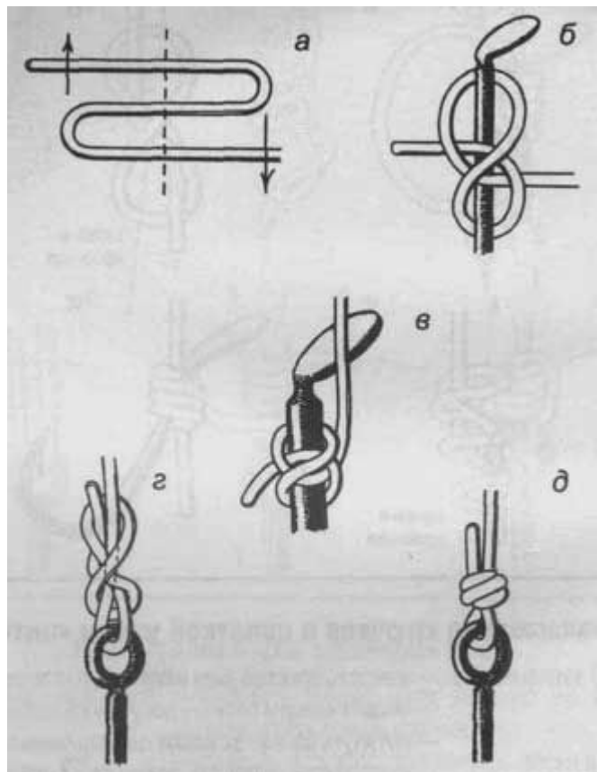
Привязывание крючков с лопаткой узлом «удавка» (а-в) Привязывание крючков с колечком узлом «питона» (г-д)
