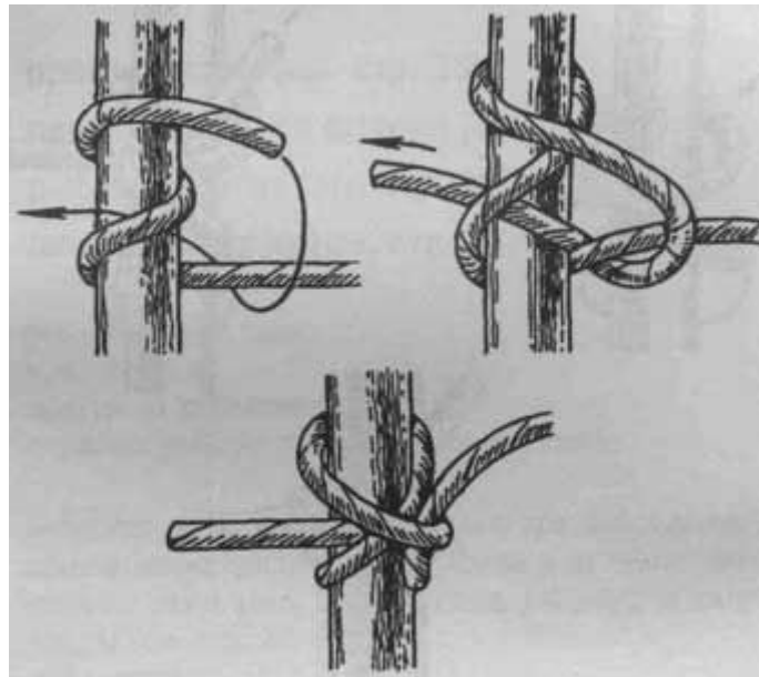
Вязание деревянного каркаса с использованием узла "питона".
