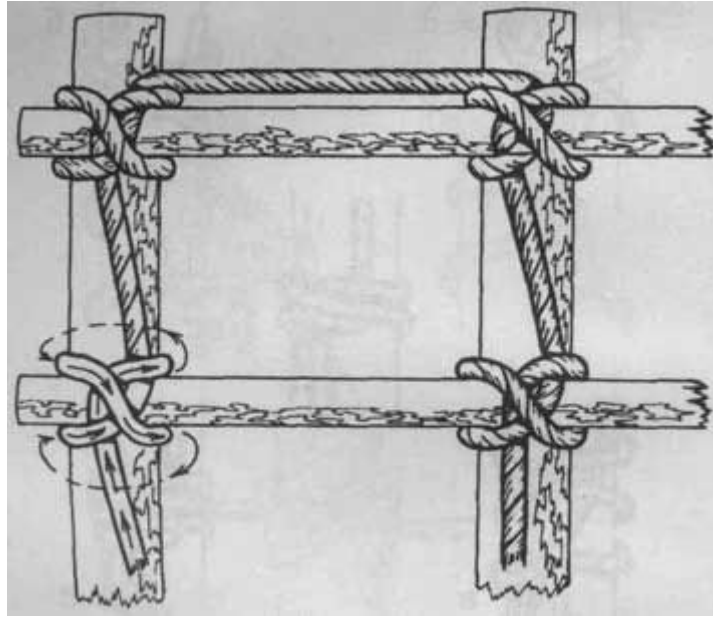
Вязание деревянного каркаса с использованием узла "питона".
